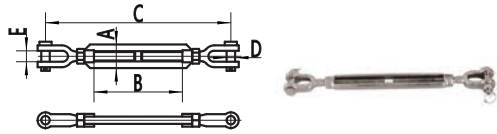
TURNBUCKLE U.S. TYPE 美式叉开体花篮
