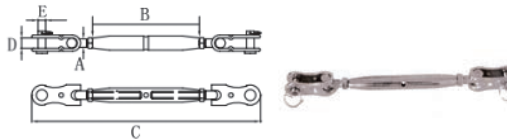
TURNBUCKLE U.S. TYPE 美式封闭叉叉花兰
