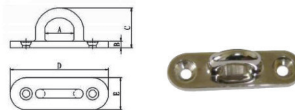
Square Eye Plate 门鼻子
