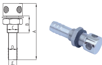
Tank Vent 透气口
