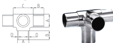
Tees 四通
