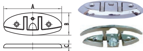
Cleat 提拉索栓
