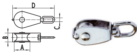
PULLEY 犁形单滑轮
