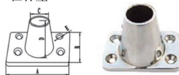
Pipe Base 栏杆座
