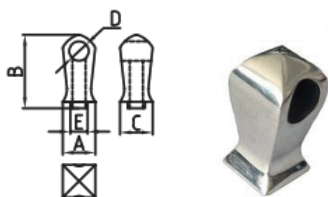
Lug 手柄
