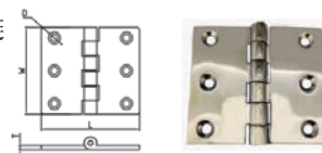
Hinge 铰链
