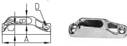
Cleats Inox For Ropes 3/6 mm 夹绳器
