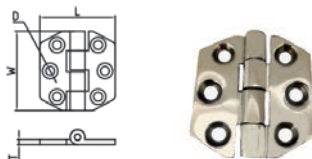
Hinge 铰链
