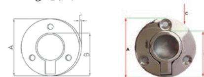
Lift Ring 地板扣
