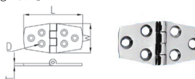
Hinge 铰链
