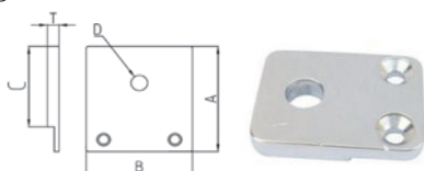
Hinge 铰链
