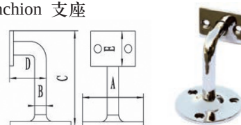
Stanchion 支座
