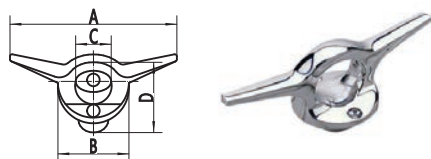
Ring Cleat 提环
