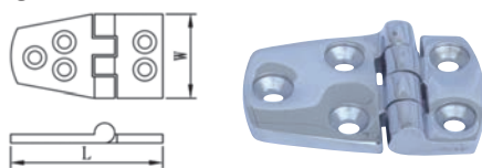
Hinge 铰链
