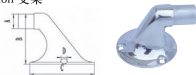
Stanchion 支架
