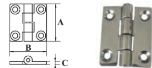
Hinge 铰链
