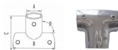
90° Tee Hand 90度三通
