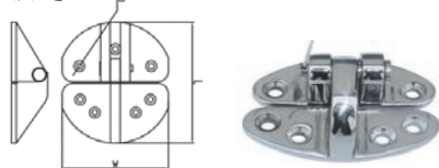
Hinge 铰链
