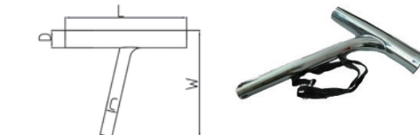
Rod Holder 鱼竿座
