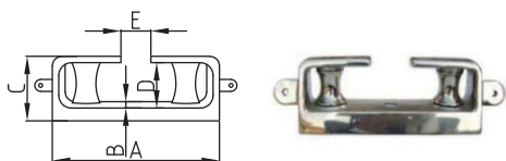
Chocks 滑轮导缆器
