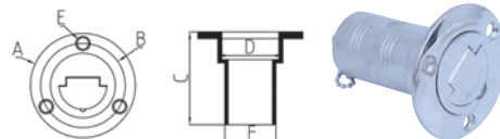
Deck filler 加油口
