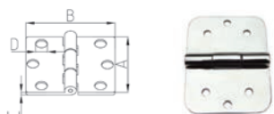
Hinge 铰链
