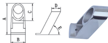
Stanchion 支架
