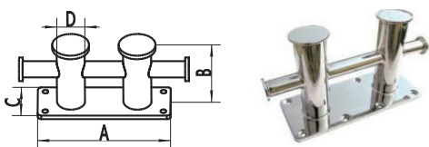
Double Cross Bollard 双十字
