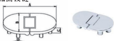
Hinge 弧面铰链
