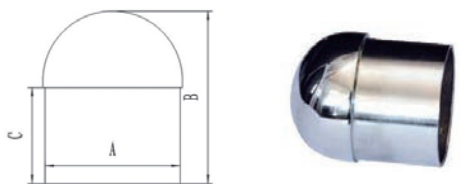
Insert 塞头
