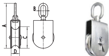
FLAT SWIVEL EYE PULLEY 方形单滑轮
