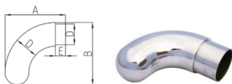
Insert 塞头
