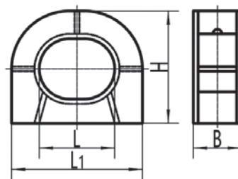
B 型 250-550
