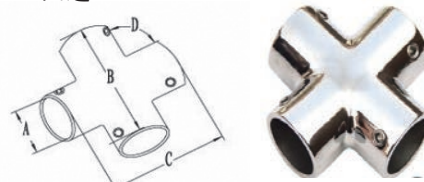
Cross 四通
