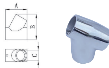
60° Tee Hand 60度三通
