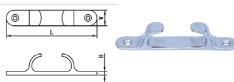
Straight chock 直导缆器
