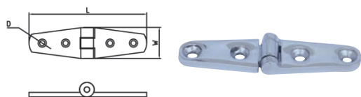
Hinge 铰链
