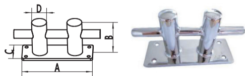
Double Cross Bollard 双十字
