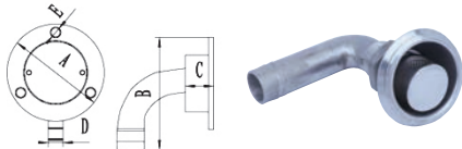
Tank Vent 透气口
