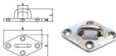
Square Eye Plate 门鼻子
