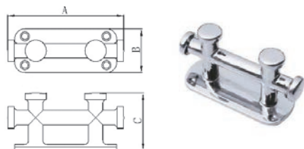
Double Cross bollard 双十字
