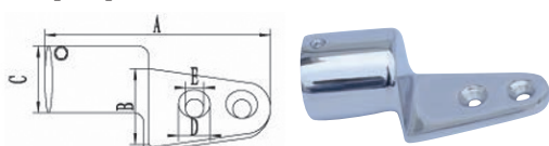
Top Cap 滑帽
