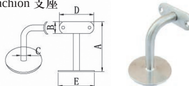
Stanchion 支座
