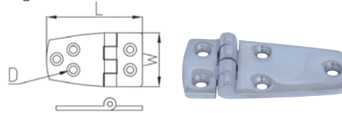
Hinge 铰链
