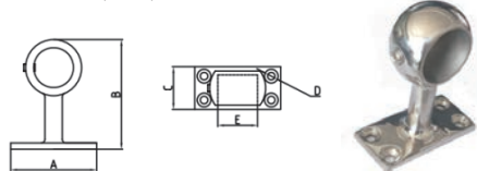
Stanchion(End) 船尾支架
