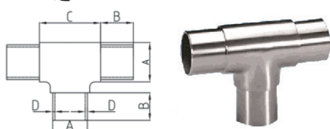
Tees 三通
