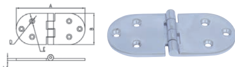
Hinge 铰链
