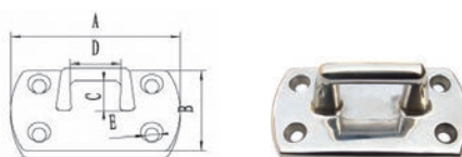
Square Eye Plate 门鼻子
