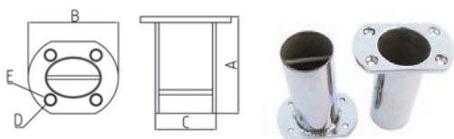
Rod Holder 鱼竿座
