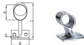
Stanchion(Center) 船中支架
