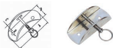
Connect Base 连接件底座
