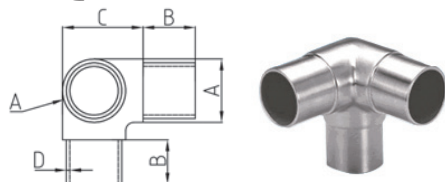
Tees 三通
